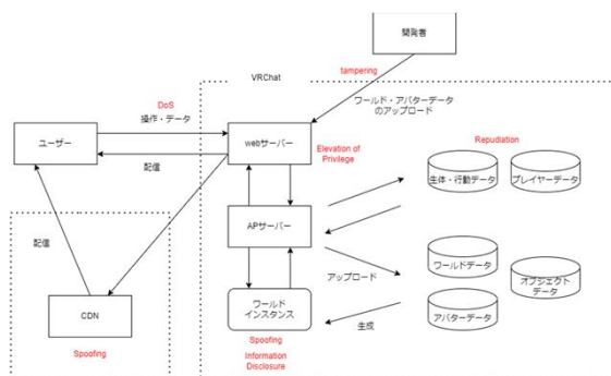
図 STRIDE分析
